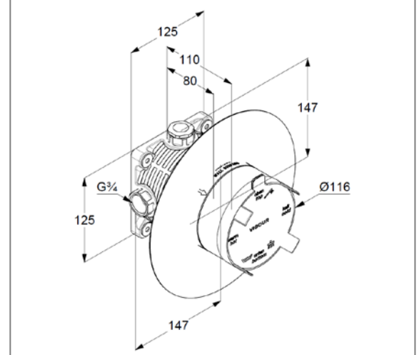
Maßzeichnung
